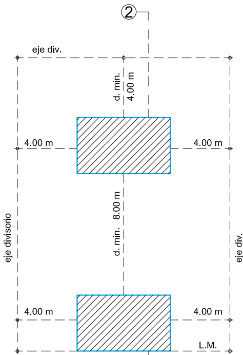
PLANTA
