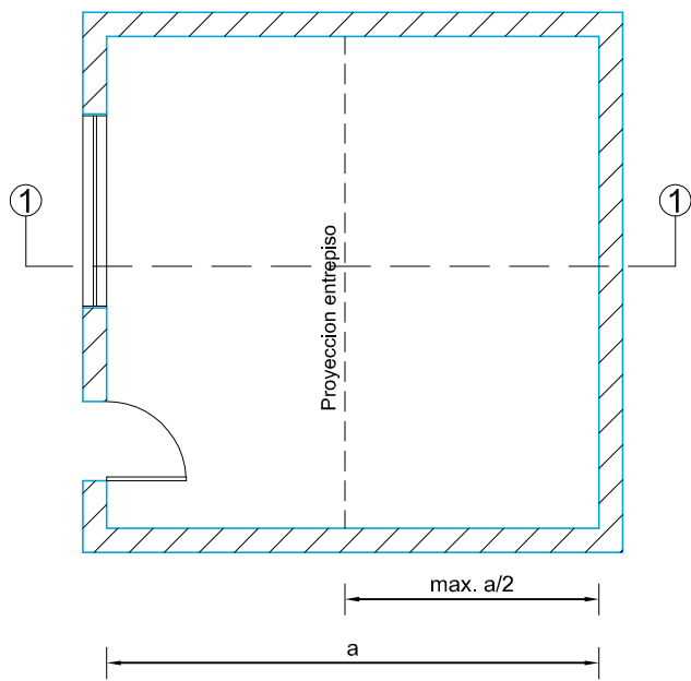
PLANTA
